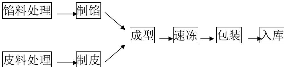
(3) 汤圆生产工艺。
