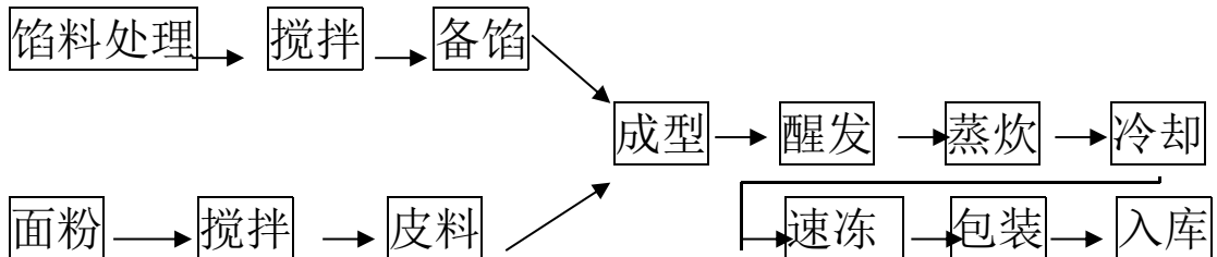
(3) 汤圆生产工艺。
